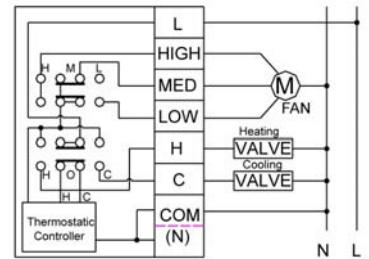
Tstat3C
