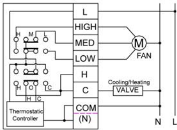
Tstat3A
